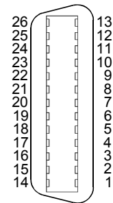
Vue de l'avant du module
